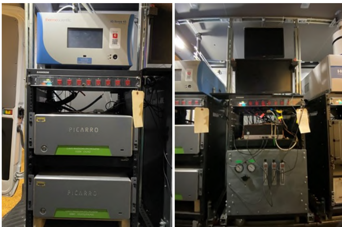
(左图)从上到下:Thermo Scientific 43iQ、Picarro G2204、Picarro G2401。(右图)从上到下: Picarro 和 Horiba 显示器，PC 显示器，带串行通信集线器的桌面工作站，泵箱
